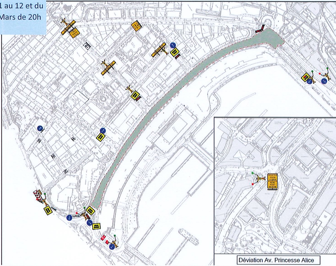
Figure 1 : Plan d'installation de chantier Bd Albert 1er
